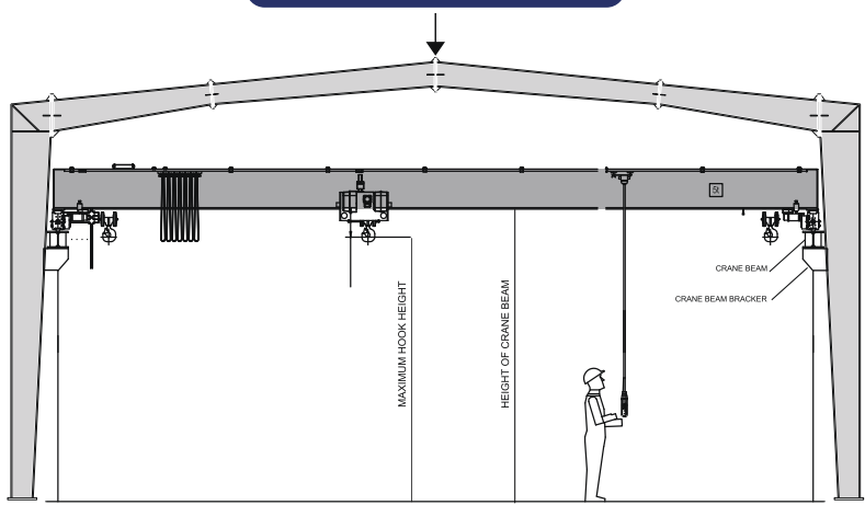
EOT Crane
